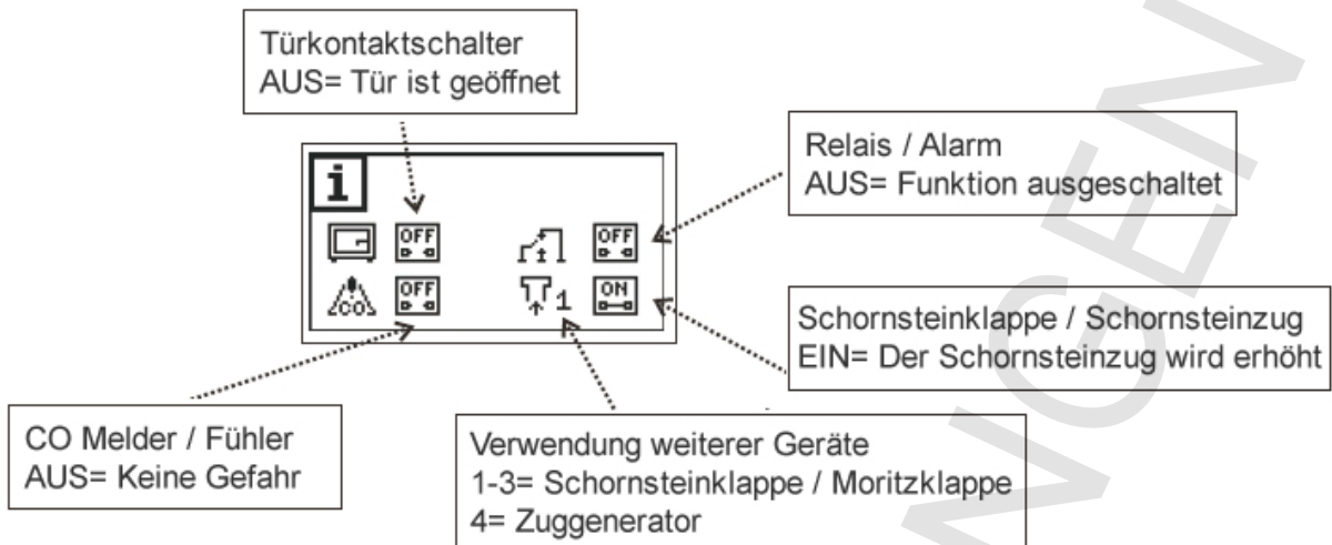
Abb. 6: Displayanzeige Anschlussinformationen
