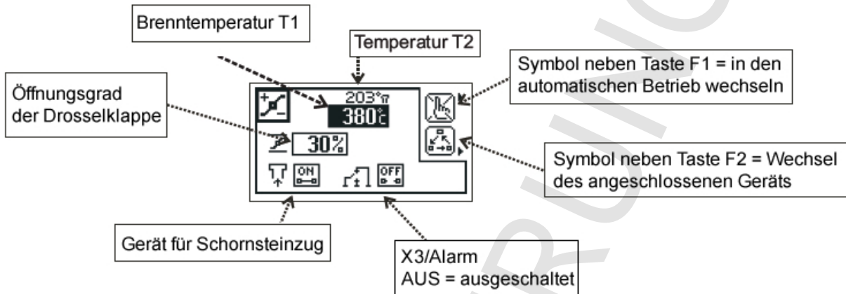
Abb. 5: Displayanzeige im manuellen Betrieb
