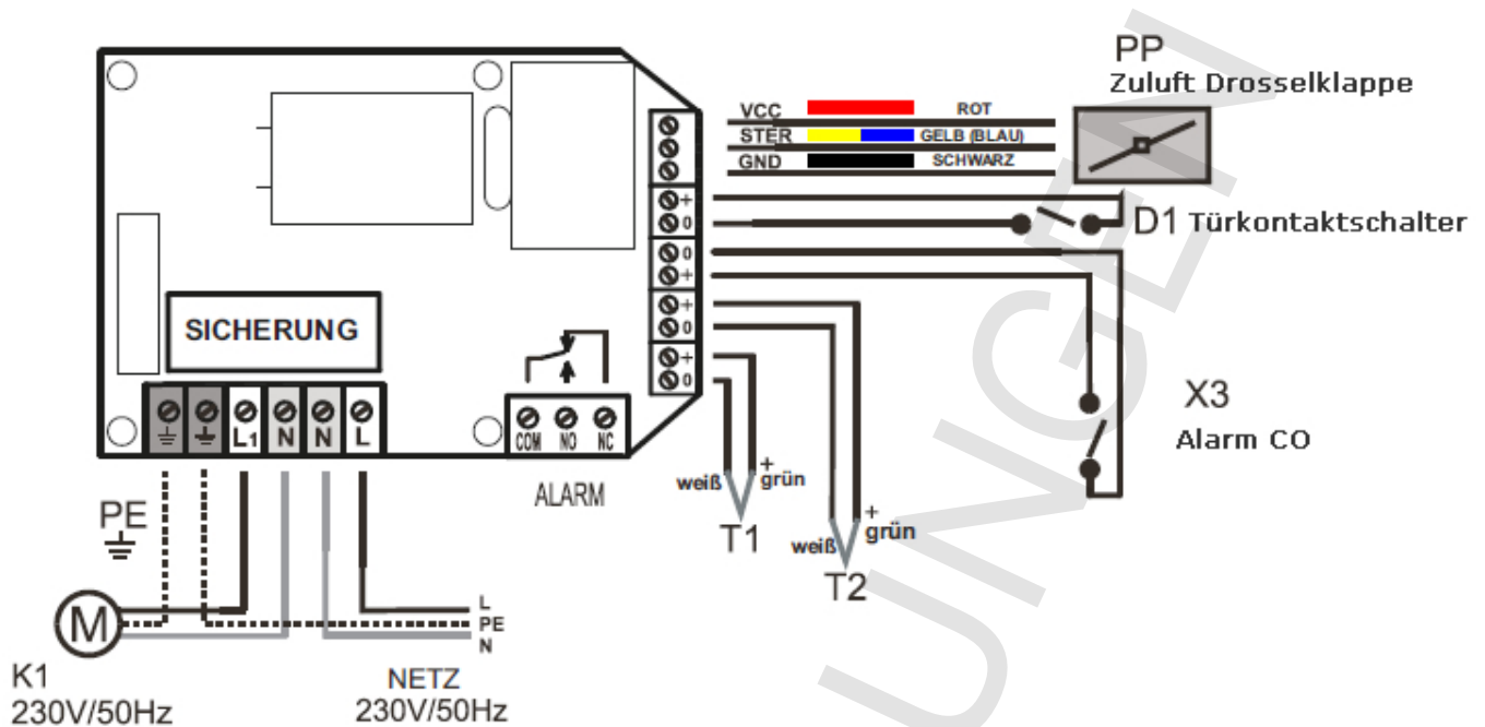
Abb. 8 – Anschlussschema der Steuerung, sowie externer Geräte
